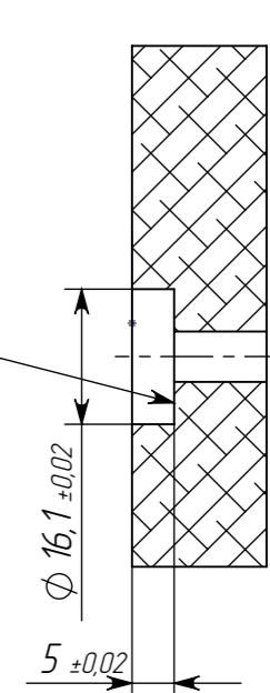
Б-Б МАСШТАБ 1:1
