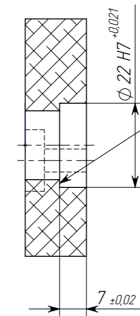
A-A МАСШТАБ 1:1
