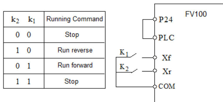
Рис 6-17. 2-х проводной рабочий режим 1
