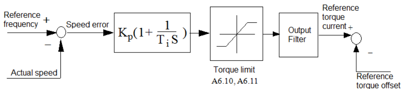
Рис. 6-13 Регулятор скорости
