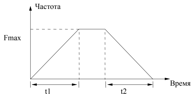
Рис. 6-12. Линейное ускорение/торможение
