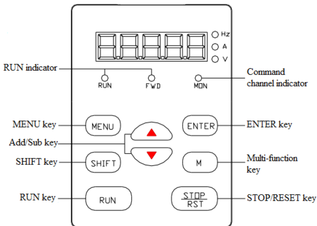
Рис. 5-1 Панель управления
