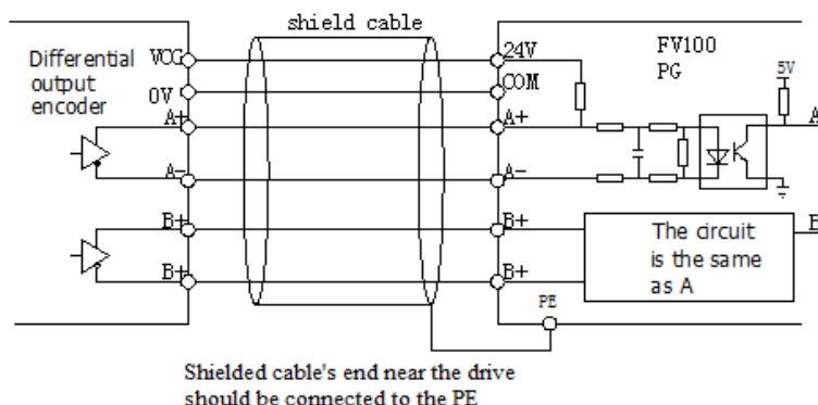
Рис 4-17 Подключение дифференциальный выход энкодера
