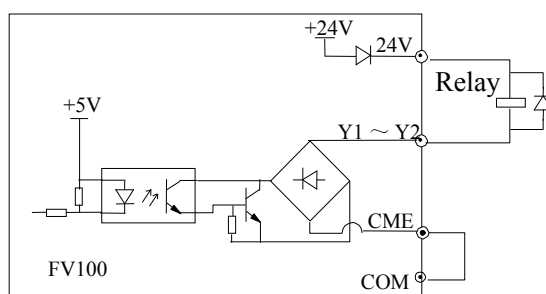
Рис. 4-13 Подключение многофункционального выхода с внутренним источником тока.
