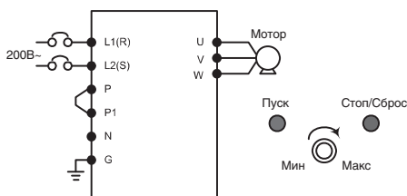
Схема подключения
