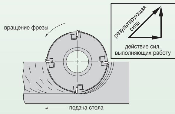
Встречное фрезерование
