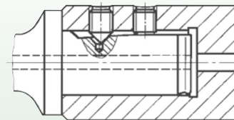
Рис. 1. Хвостовик сверла по DIN 6595/ISO 9766 и крепление с помощью винтов с коническим и плоским торцем.
