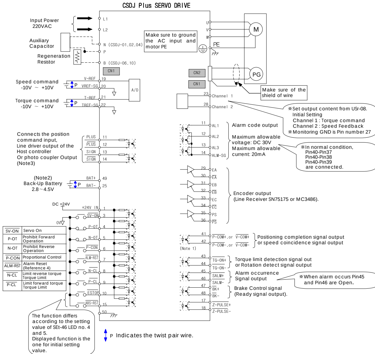
Fig 2.9 Wiring
