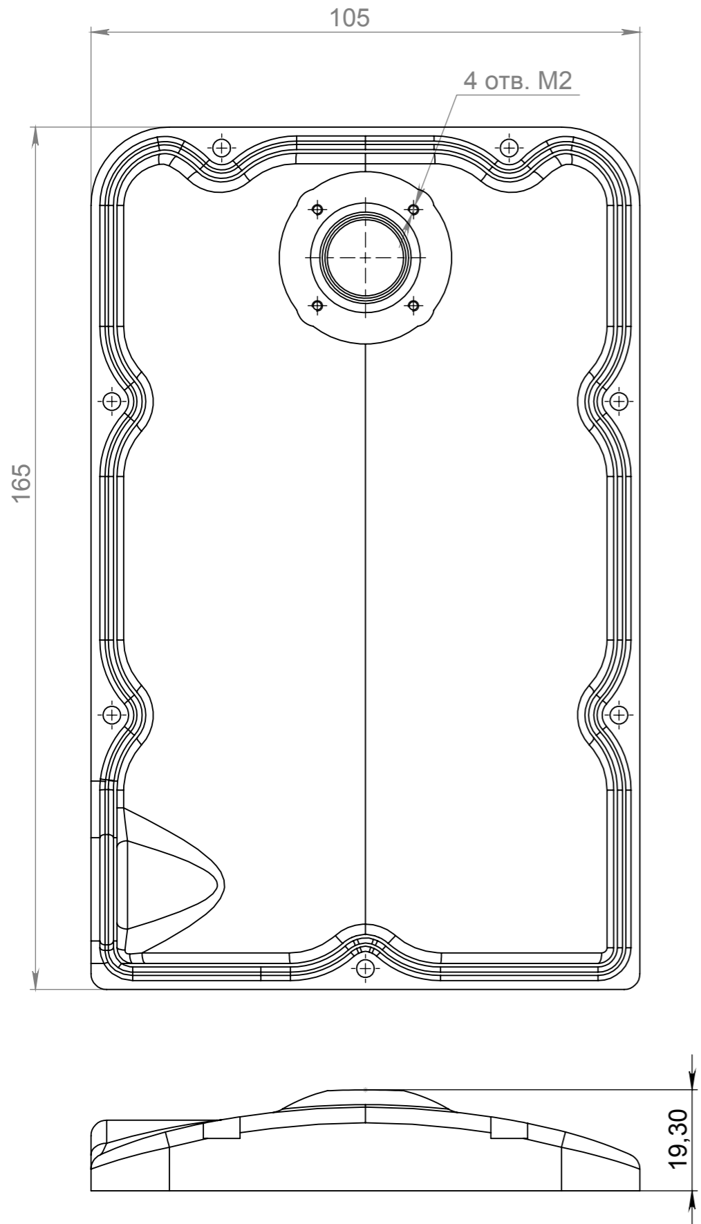
001_MetallHousing_v1_front
