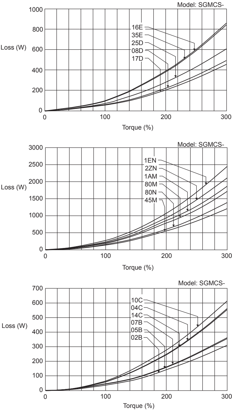
(d) SGMCS servomotor
