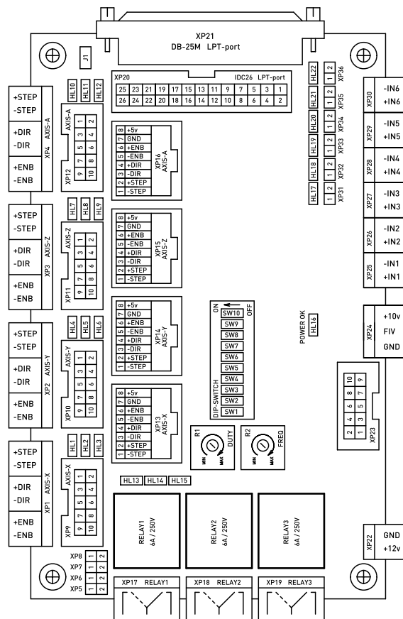
Рис. 2. Подключение модуля
