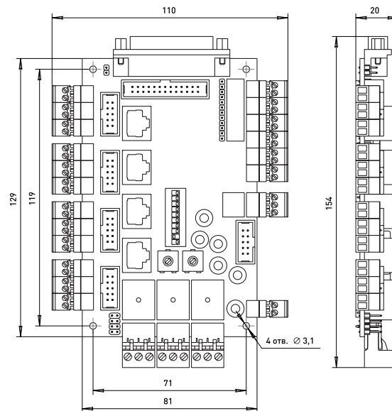
Рис. 1. Размеры устройства коммутации PLC4x-G2
