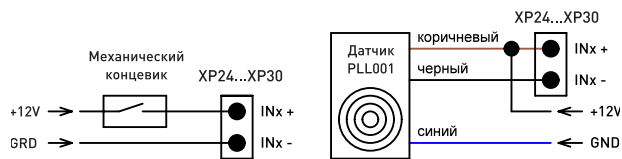
Рис. 4. Подключение концевых датчиков
