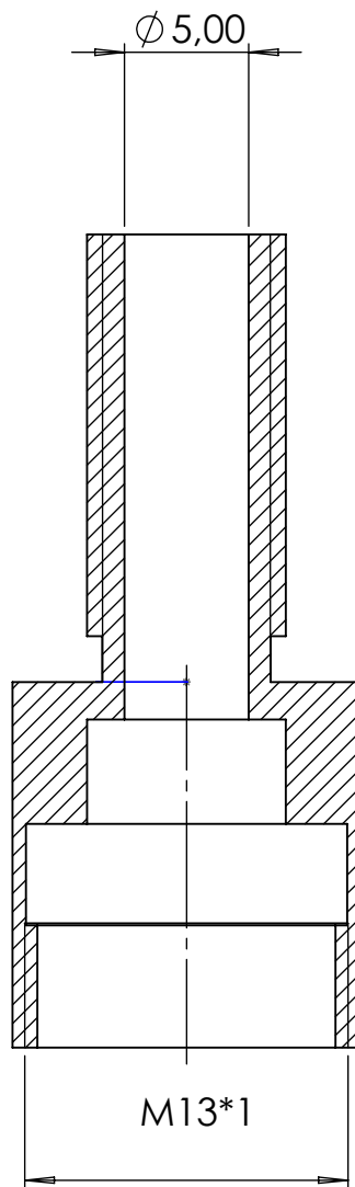
СЕЧЕНИЕ А-А МАСШТАБ 3 : 1
