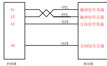
步进电机差分接法
