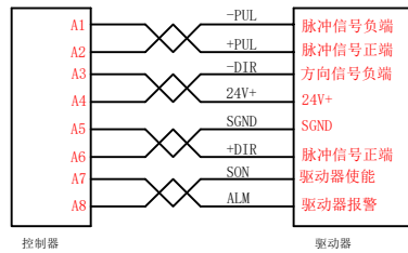
伺服电机接法1不接反馈
