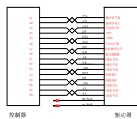
伺服电机接法2带反馈
