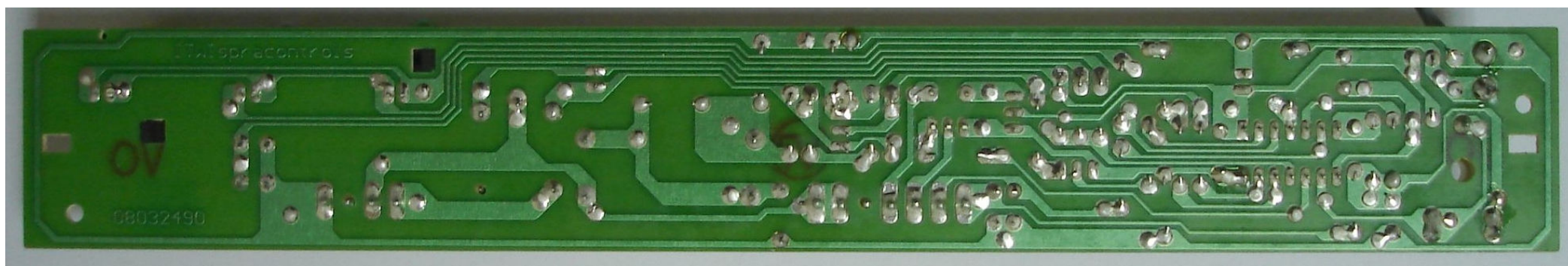
Плата управления холодильника ARDO CO 3012 SA. Вид со стороны монтажа, плата перевернута относительно горизонтальной оси.
