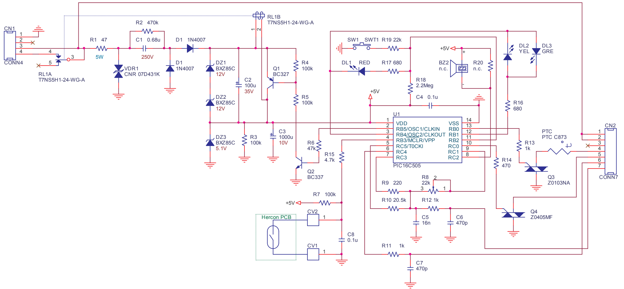
Электрическая схема платы управления холодильника ARDO CO 3012 SA.
