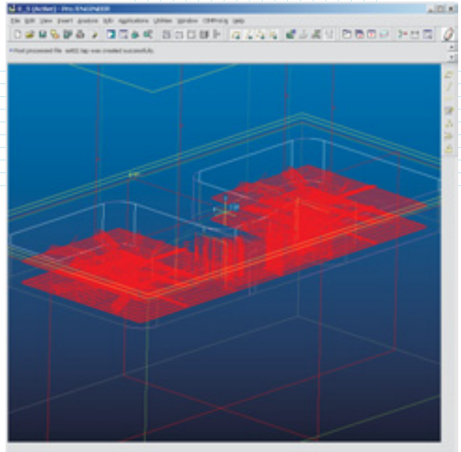
Рис. 25. Траектория для обработки с большой глубиной резания
