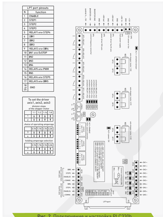
Рис. 2. Подключение и настройка PLC330b
