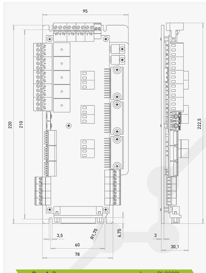
Рис. 1. Размеры многоканального драйвера PLC330b
