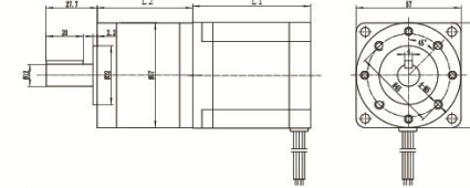
PL57-B 外形图 (Dimensions) (单位/unit=mm)
