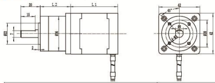
PL42-B 外形图 (Dimensions) (单位/unit=mm)
