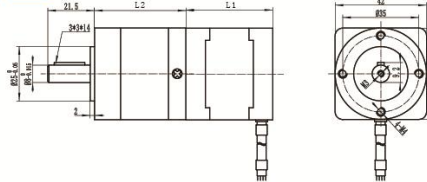
PL42 外形图 (Dimensions) (单位/unit=mm)
