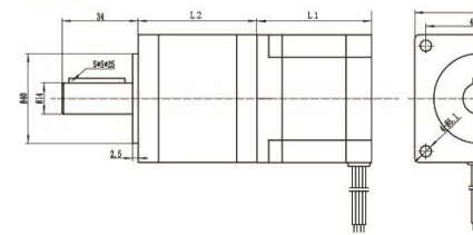
PL57 外形图 (Dimensions) (单位/unit=mm)
