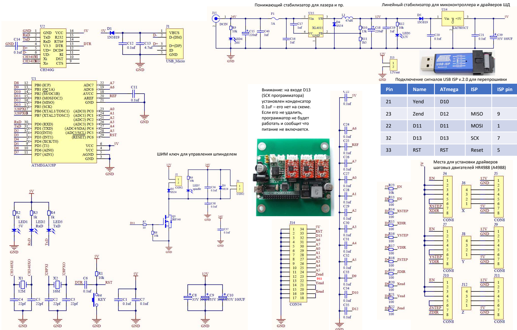
Принципиальная схема контроллера китайских гравировальных станков CNC3018 и CNC1610 Woodpecker GRBL 0.9
