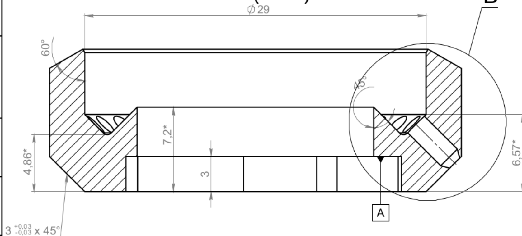
A-A (5 : 1)
