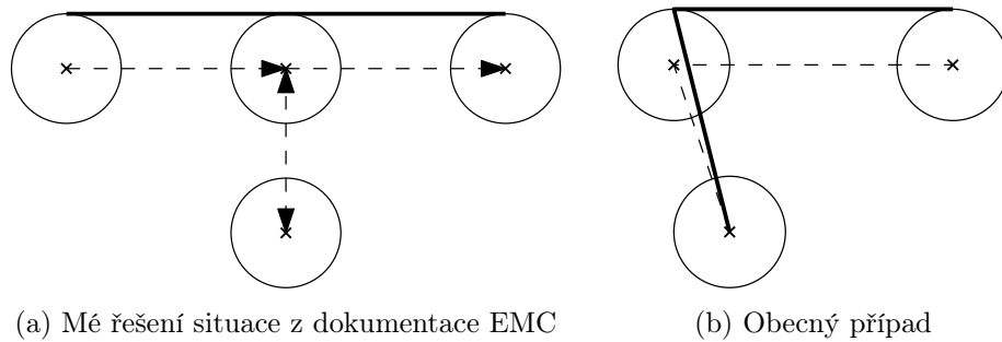
Obrázek 8.5: Implementace lineárního lead-in pohybu v mém systému. Tlustá čára znázorňuje trasu zadanou G-kódem, přerušovaná pak dopočtenou korekci.
