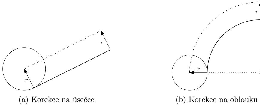
Obrázek 8.2: Znázornění základní korekce. Černou čarou je znázorněna naprogramovaná kontura (tedy trasa zadaná G-kódem), přerušované pak dopočtená korigovaná trasa.
