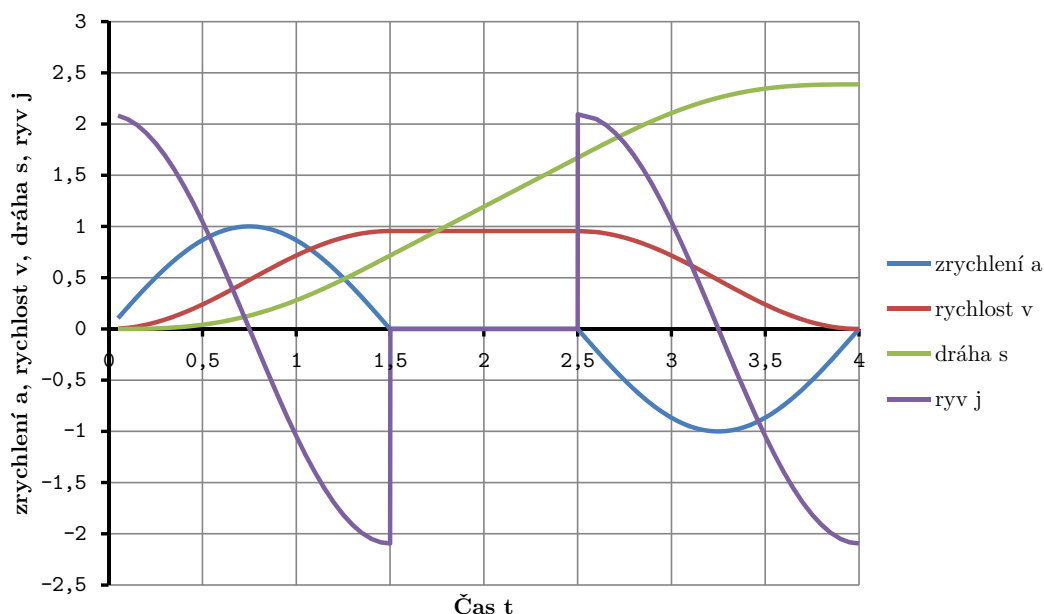
Obrázek 5.1: Graf znázorňující průběh jednotlivých veličin při použití sinového zrychlení. Je složen z 1,5 sekundového rozjezdu z rychlosti v_0 = 0 ; 2 sekundového pohybu přímočarého a 1,5 sekundového brždění na nulovou rychlost.
