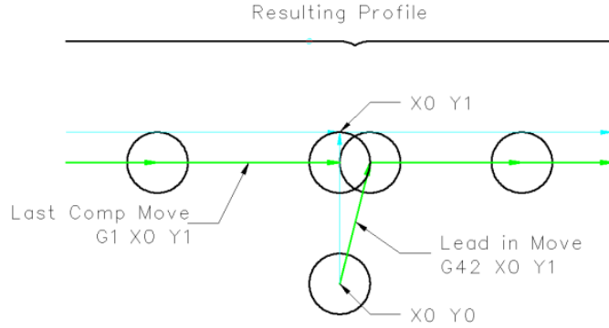
Obrázek 8.4: Implementace chování lineárního lead-in pohybu v systému EMC. Převzato z < http://www.linuxcnc.org/docs/2.4/html/comp02.png >
