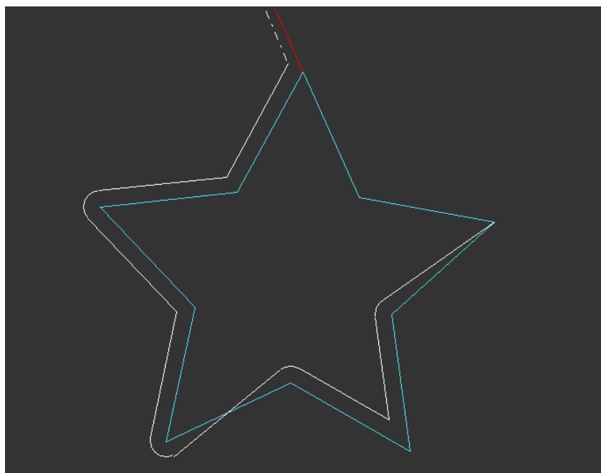
Obrázek 8.8: Ukázka zpracování korekce průměru nástroje mým systémem.
