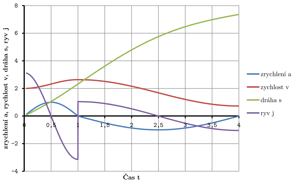
Obrázek 5.2: Graf znázorňující průběh jednotlivých veličin při použití sinového zrychlení. Je složen ze sekundového rozjezdu z rychlost v_0 = 1 a 2 sekundového brždění na brzdou rychlost v_b
