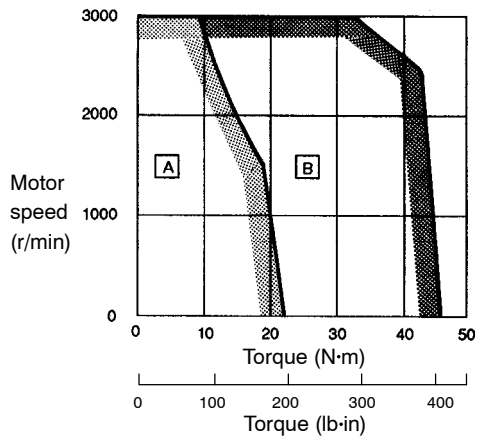
SGMG-30A □A
