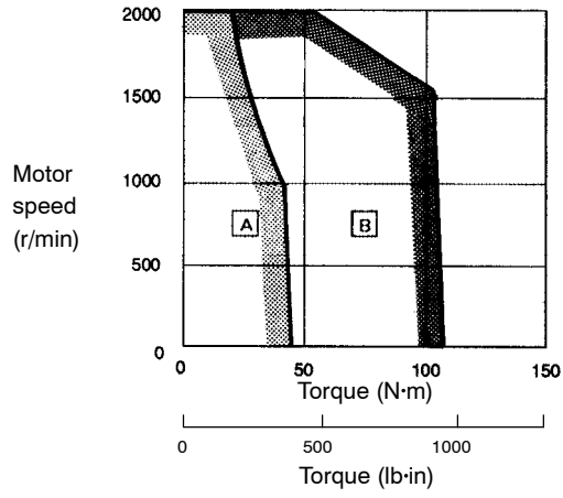
SGMG-44A□B
