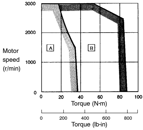
SGMG-55A □ A
