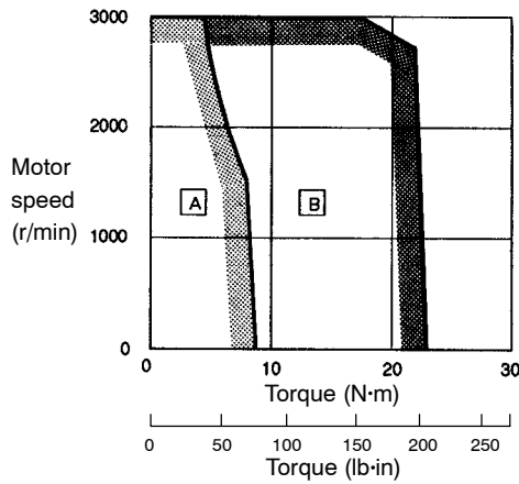
SGMG-30A □A
