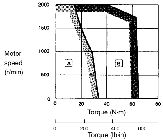
SGMG-30A□B
