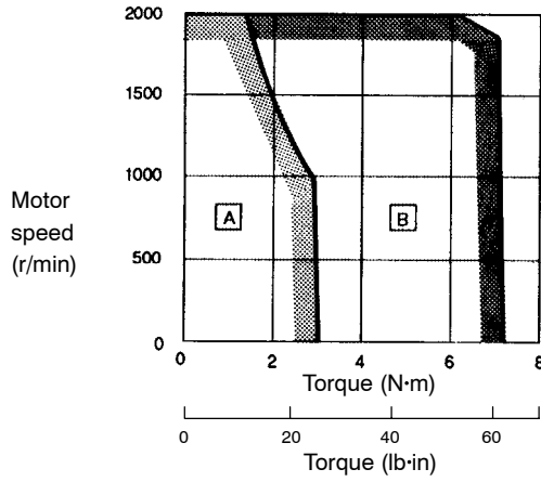
SGMG-09A□B
