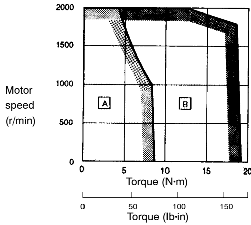
SGMG-09A□B
