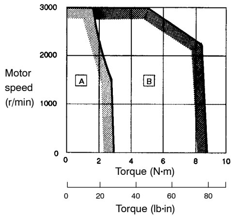
SGMG-13A □A
