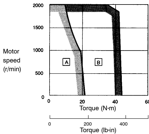
SGMG-20A□B
