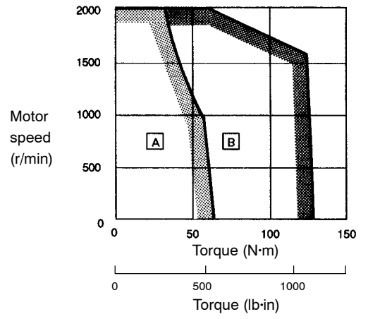
SGMG-60A□B
