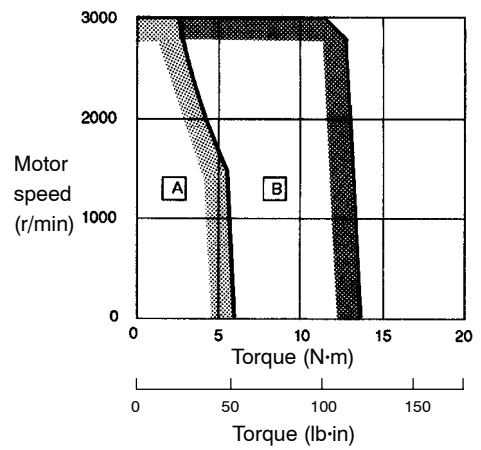
SGMG-20A □A
