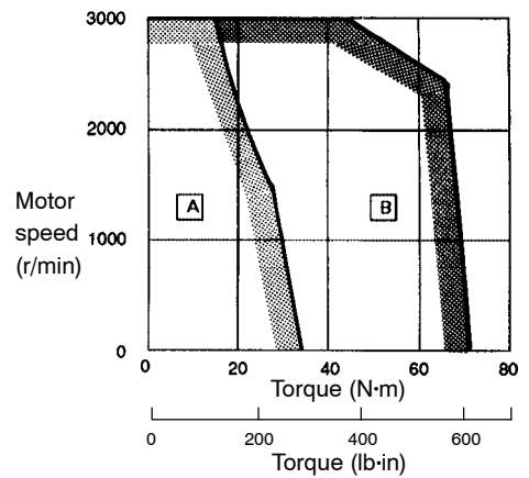
SGMG-44A □A
