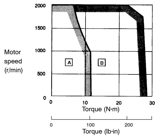
SGMG-12A□B
