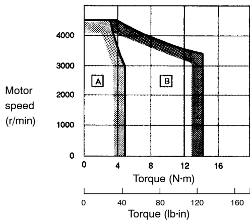
SGMP-15A
