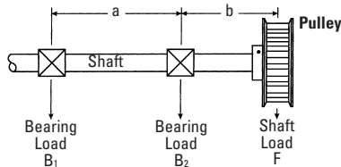
Fig. 31 Overhung Pulley
