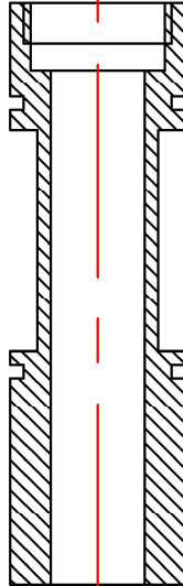
втулка лінзотримач
