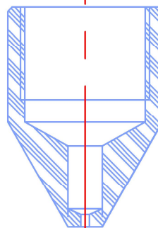
сопло регулювання
